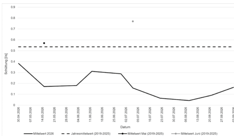
Wasserführung einer Quelle in der Val Ftur in Schweizerischen Nationalpark. (Grafik: Nicola Steiner)
